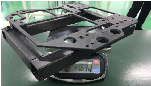
CFRP治具の例（エンジン搬送用）
